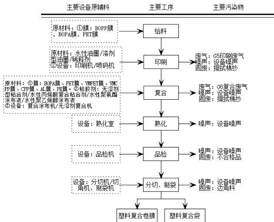
图 3-3 1号厂房塑料复合卷膜、袋生产工艺流程及产污环节
