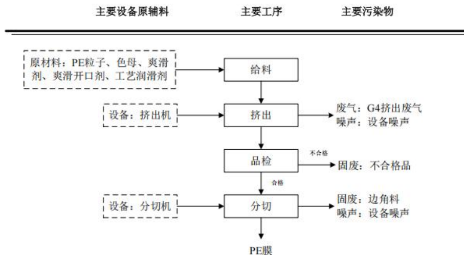
图 3-2 PE 膜生产工艺流程及产污环节
